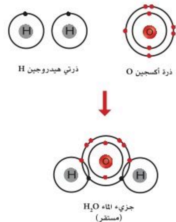
الشكل ب٦ الرابطة التساهمية القطبية في جزيء الماء H_2O .
