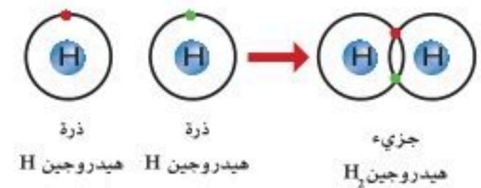
الشكل أ٦ الرابطة التساهمية غير القطبية في جزيء الهيدروجين H_2 .
